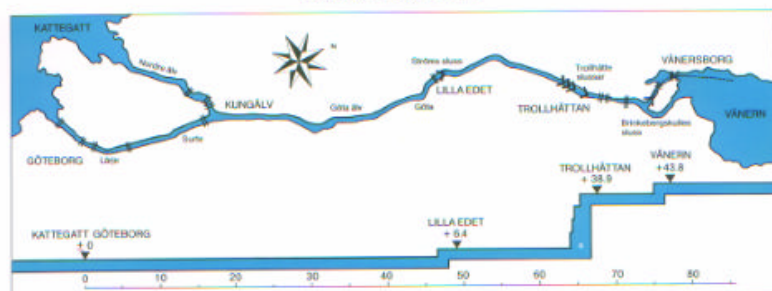
Bilden visar hur nivåskillnaden mellan Vänern och Västerhavet fördelas på de sex slussarna.
